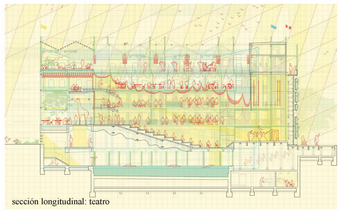
sección longitudinal: teatro
